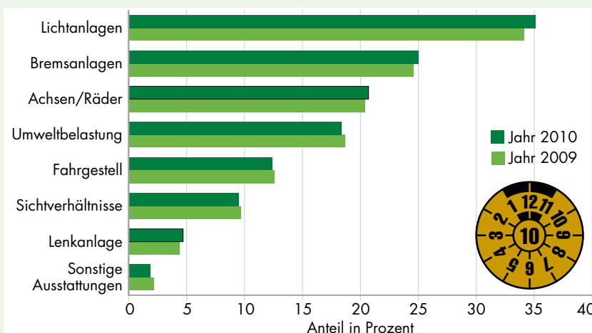
31 Ergebnisse der Pkw-Untersuchungen 2010 – Pkw nach Mängelarten
